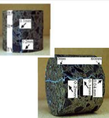
裂縫鑽心取樣
