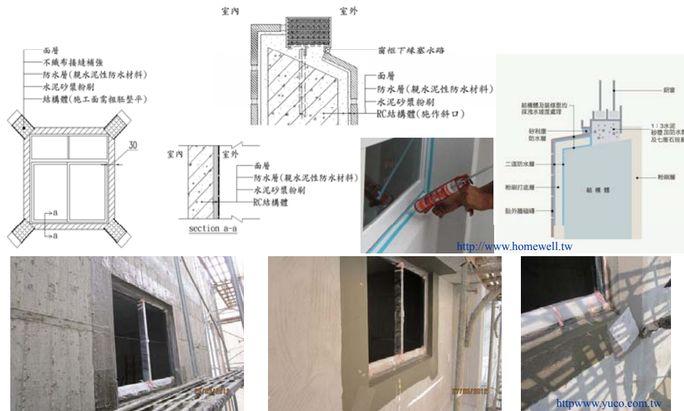
窗框結構體第一道防水
